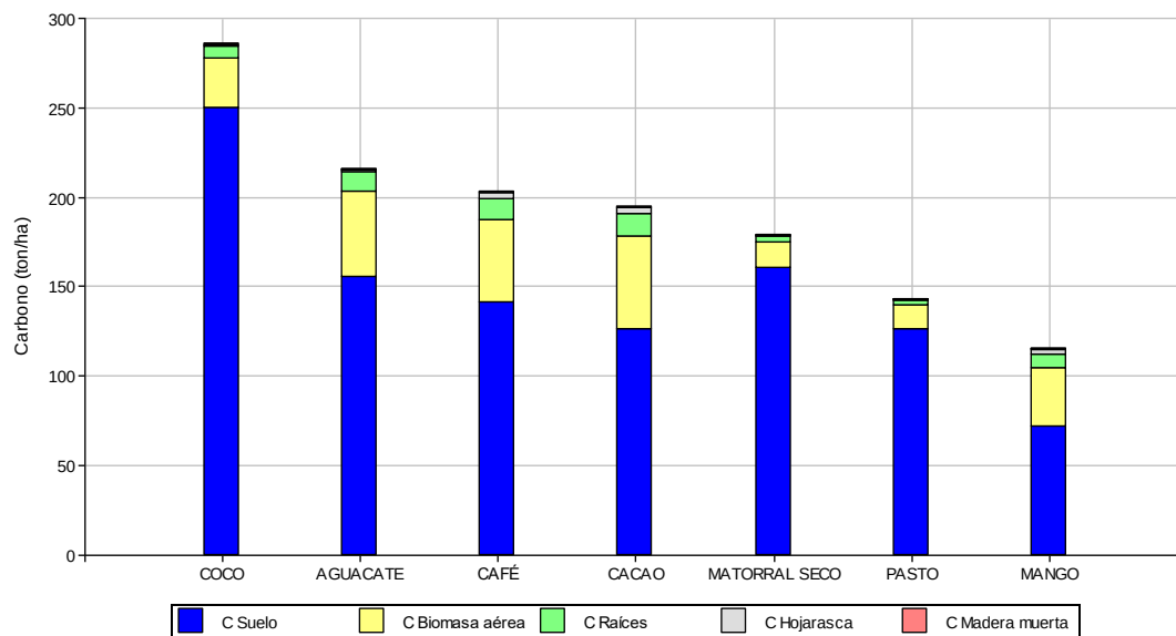
Figura 3. Comparación del carbono almacenado, por componente, entre plantaciones de cobertura No Bosque, República Dominicana (2018)
