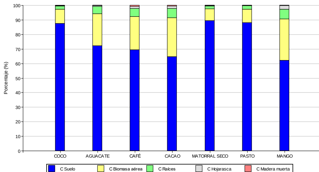
Figura 4. Comparación del porcentaje de carbono almacenado, por componente, entre plantaciones de cobertura No Bosque, República Dominicana (2018)
