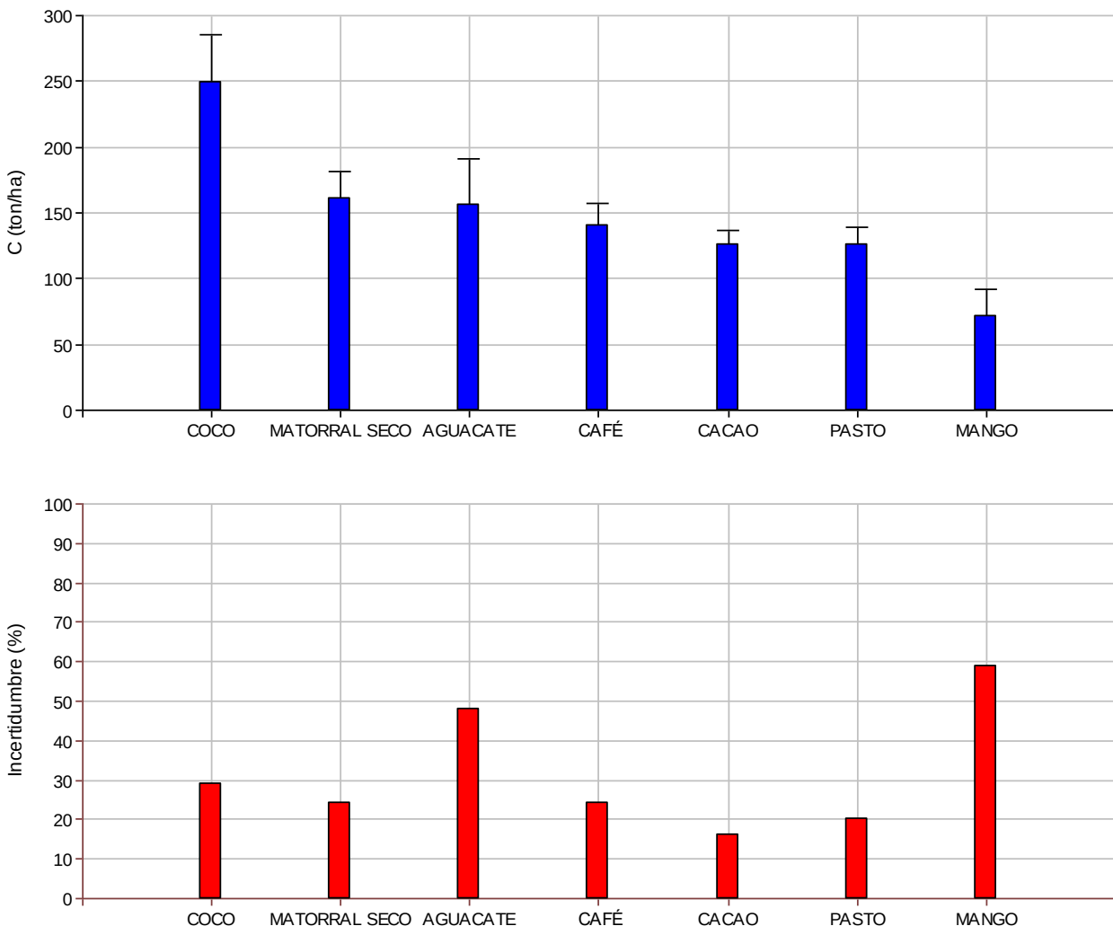
Figura 5. Comparación del carbono almacenado (medias y error estándar) e incertidumbre de la estimación en el suelo, entre plantaciones de cobertura No Bosque, República Dominicana (2018)
