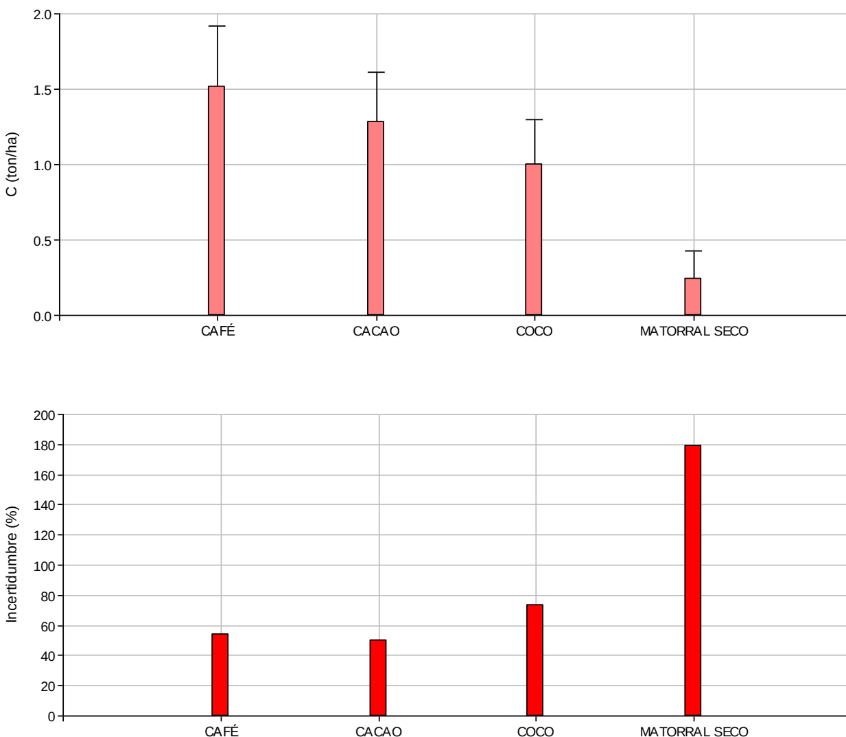
Figura 9. Comparación del carbono almacenado (medias y error estándar) e incertidumbre de la estimación en la madera muerta, entre plantaciones de cobertura No Bosque, República Dominicana (2018)
