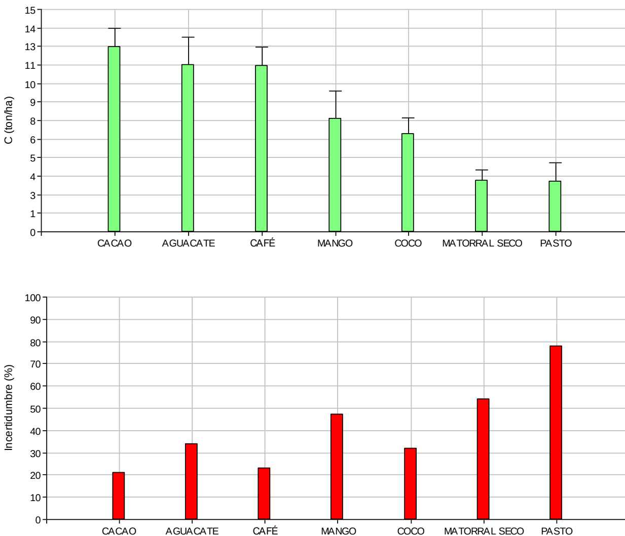
Figura 7. Comparación del carbono almacenado (medias y error estándar) e incertidumbre de la estimación en las raíces, entre plantaciones de cobertura No Bosque, República Dominicana (2018)
