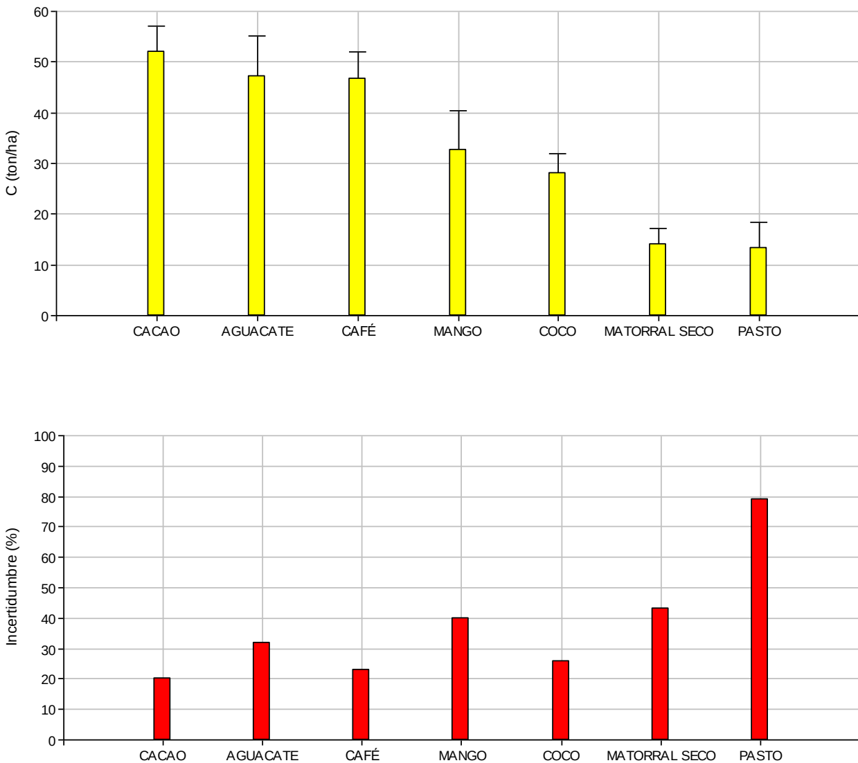
Figura 6. Comparación del carbono almacenado (medias y error estándar) e incertidumbre de la estimación en la biomasa aérea, entre plantaciones de cobertura No Bosque, República Dominicana (2018)
