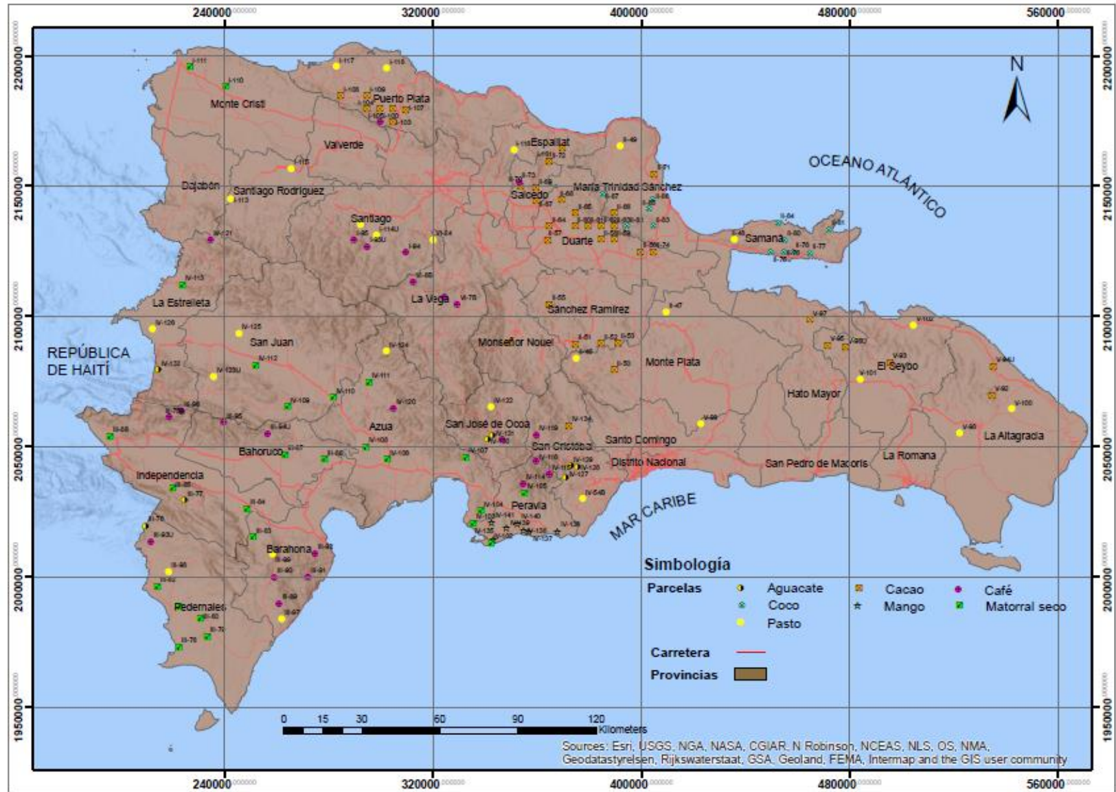
Figura 2. Ubicación de las 142 unidades de muestreo inventariadas y analizadas para la estimación de biomasa, carbono y CO 2eq en República Dominicana (2018)
