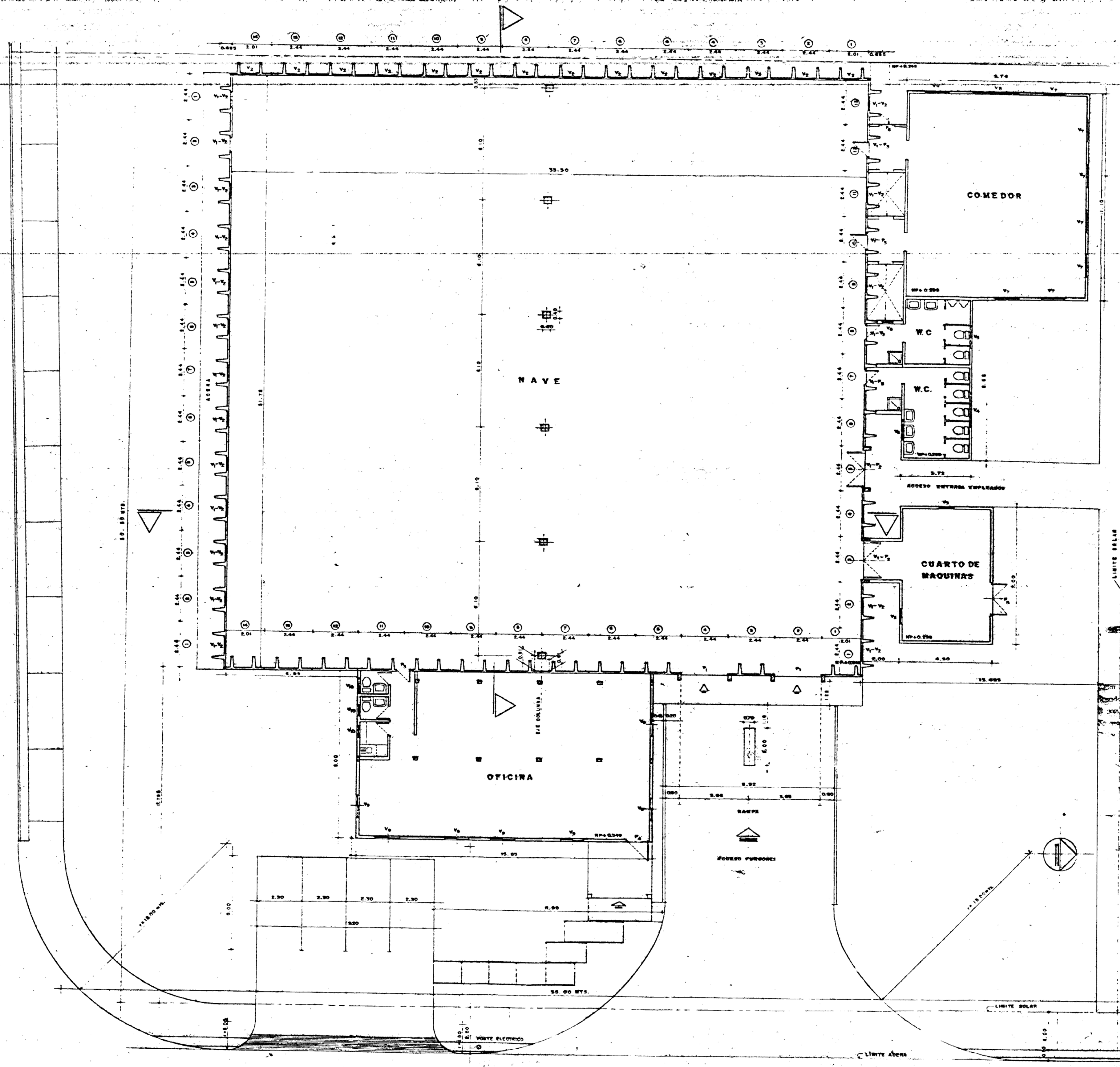
PLANTA ARQUITECTONICA NAVE... ESC. 1:100
