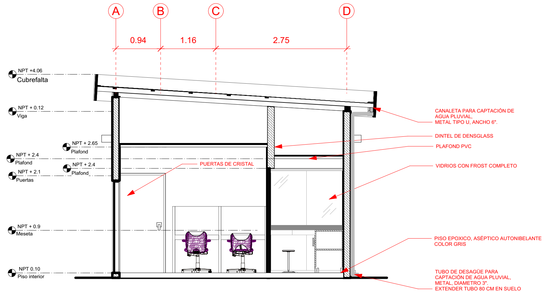
1 SECCIÓN B-B' Scale: 1:50
