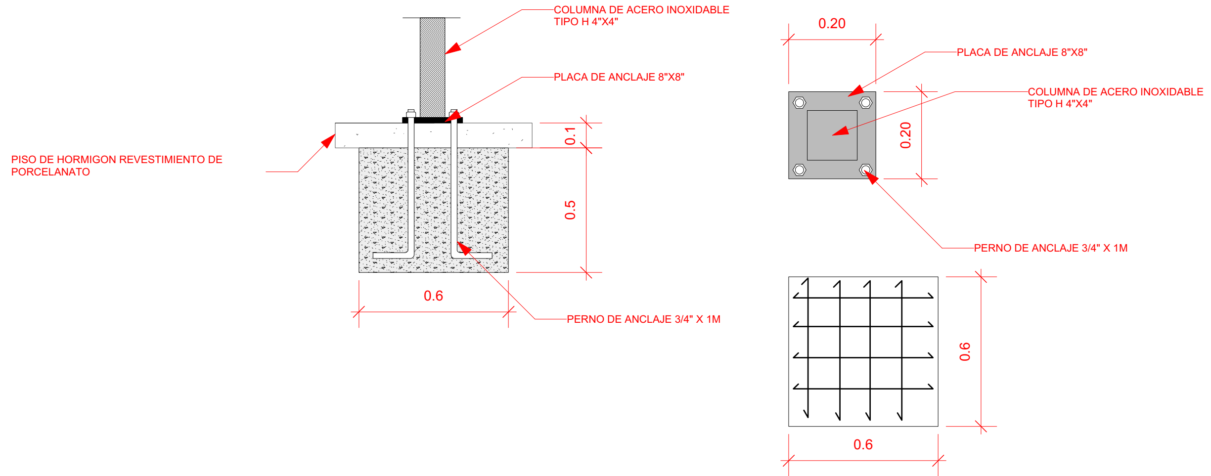
1 DETALLE ESTRUCTURAL Scale: 1:15
