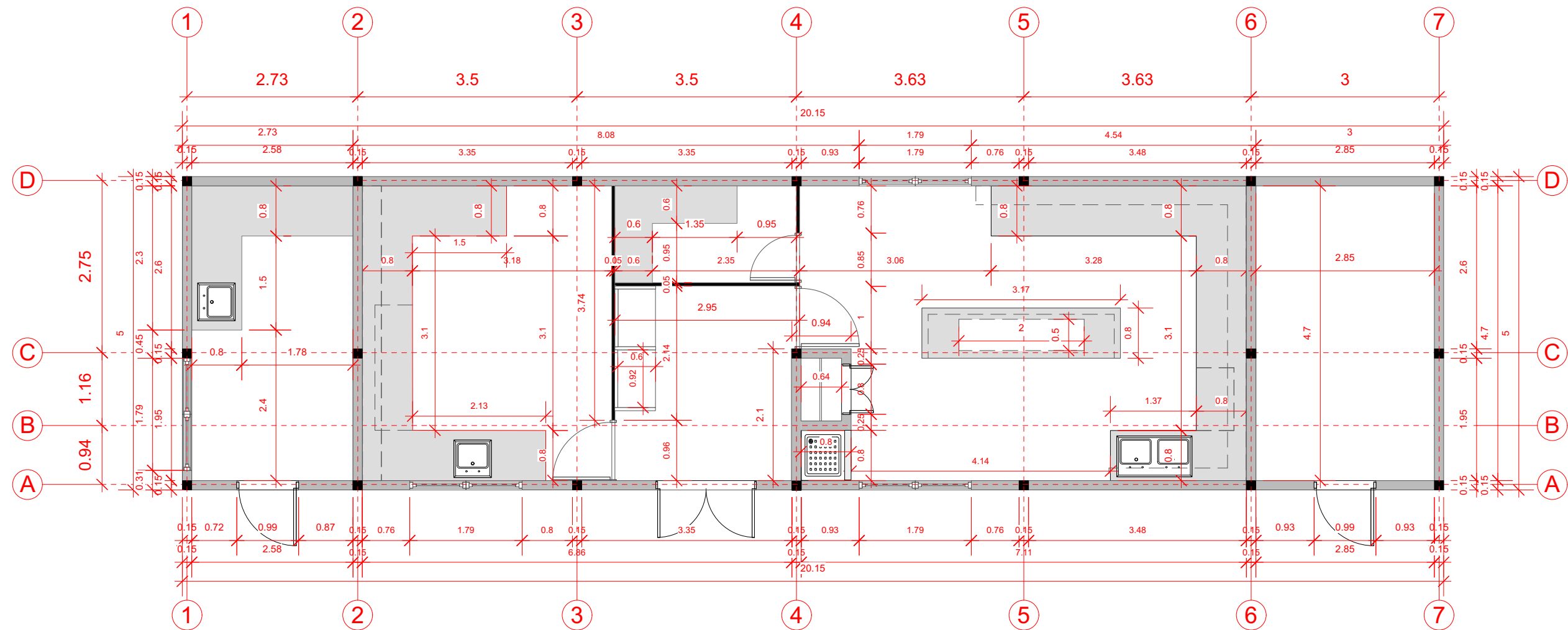
1 PLANTA DIMENSIONADA Scale: 1:75
