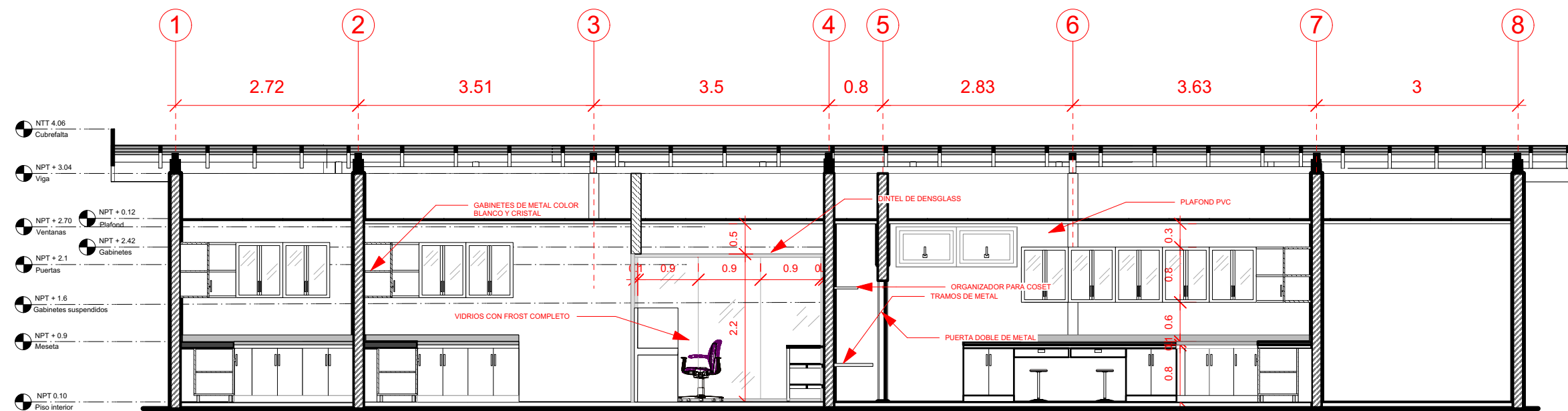
1 SECCIÓN A-A' Scale: 1:75
