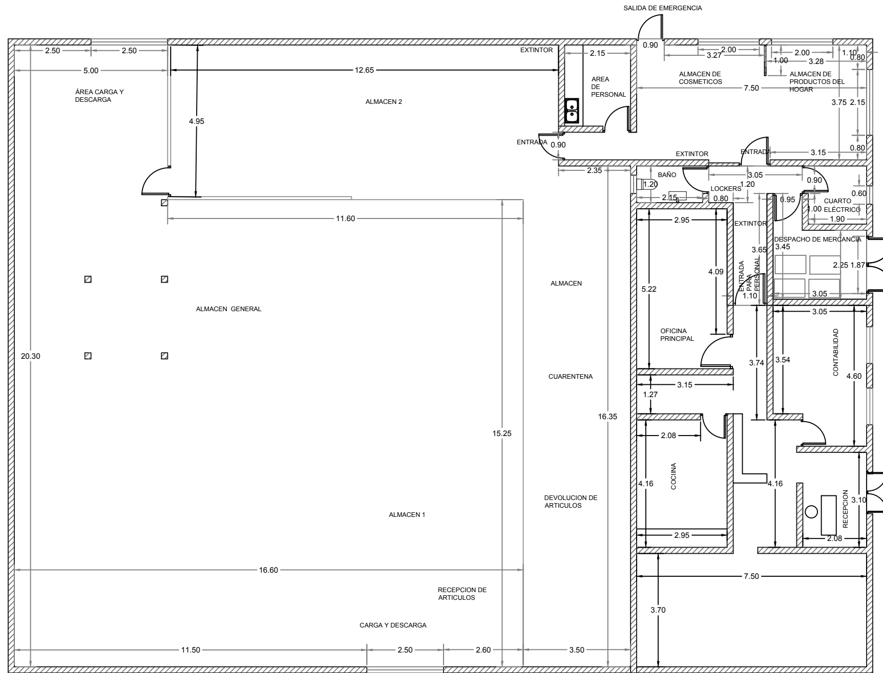
2.1 PLANTA ARQUITECTÓNICA DIMENSIONADA UPSY MULTIMARCAS S.R.L. ESC:1:150
