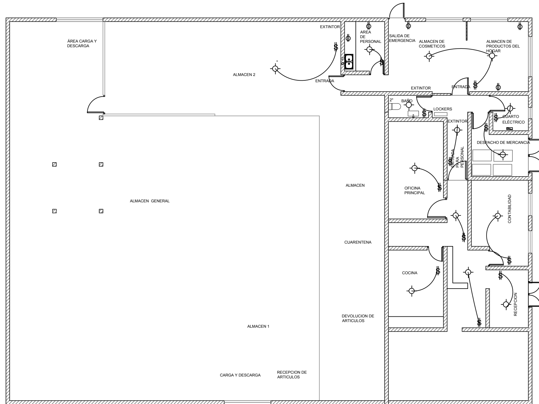
4.1 PLANTA ELÉCTRICA UPSY MULTIMARCAS S.R.L. ESC:1:150
