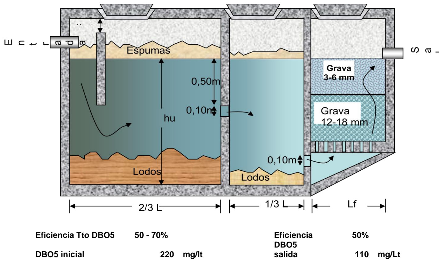
Figura # 4.- Esquema general PTAR FAFA
