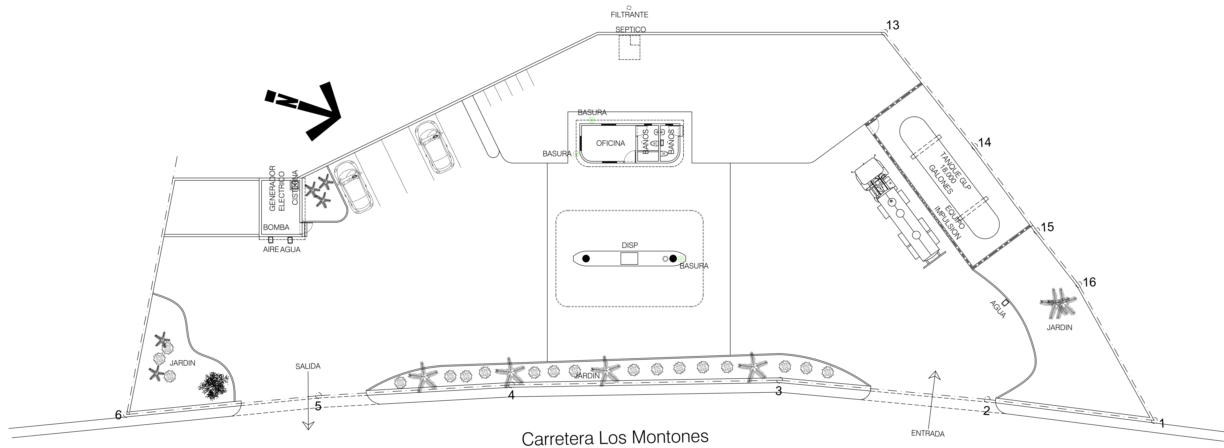
1 A4 PLANTA CONJUNTO AMUEBLADA Y PLANTA DE PLAFON MARQUESINA ESC.: 1:150 AREA: 1904.95 m2
