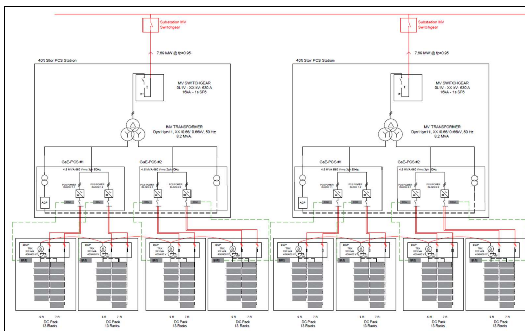
Figura 3: Esquema unifilar del sistema BESS
