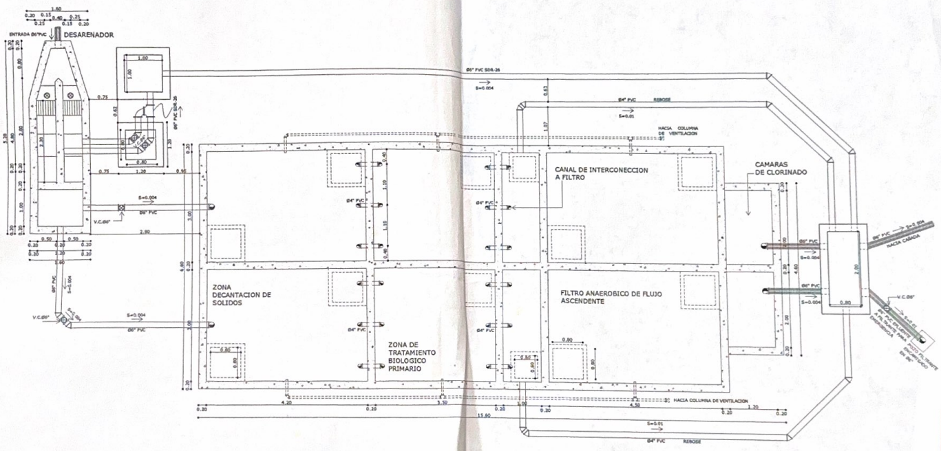
• PLANTA ARQ. PLANTA DE TRATAMIENTO No escala
