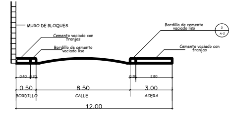
2 DETALLE CALLE CIRCULACION INTERNA A-2 NO ESCALA
