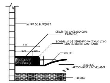
3 DETALLE BORDILLO A-2 NO ESCALA
