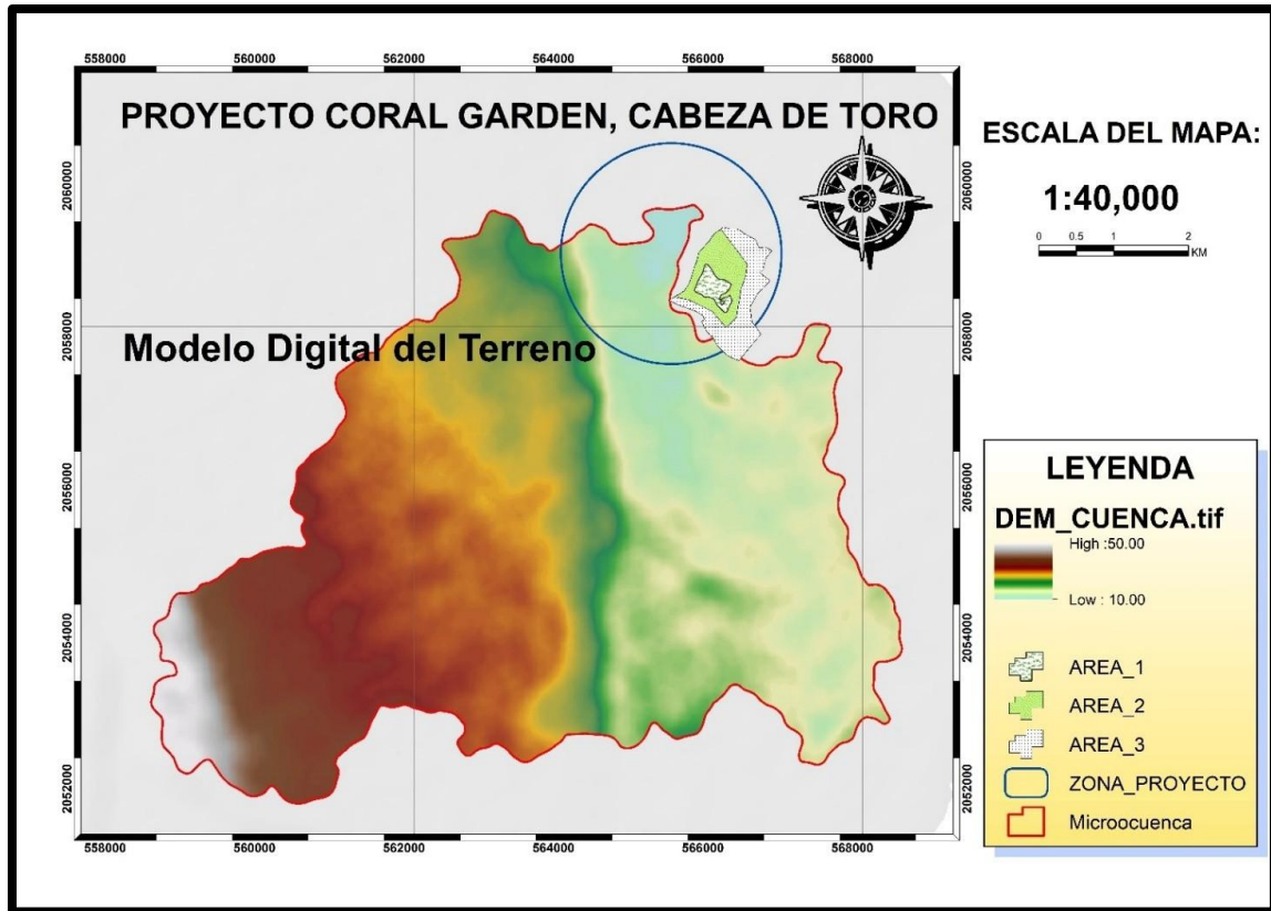
Modelo Digital del Terreno (MDT), delimitación del área de estudio y el proyecto
