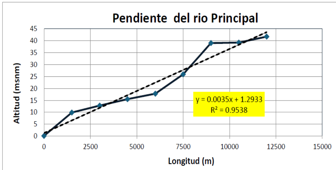
Gráfico N° 04: Pendiente del río Principal
