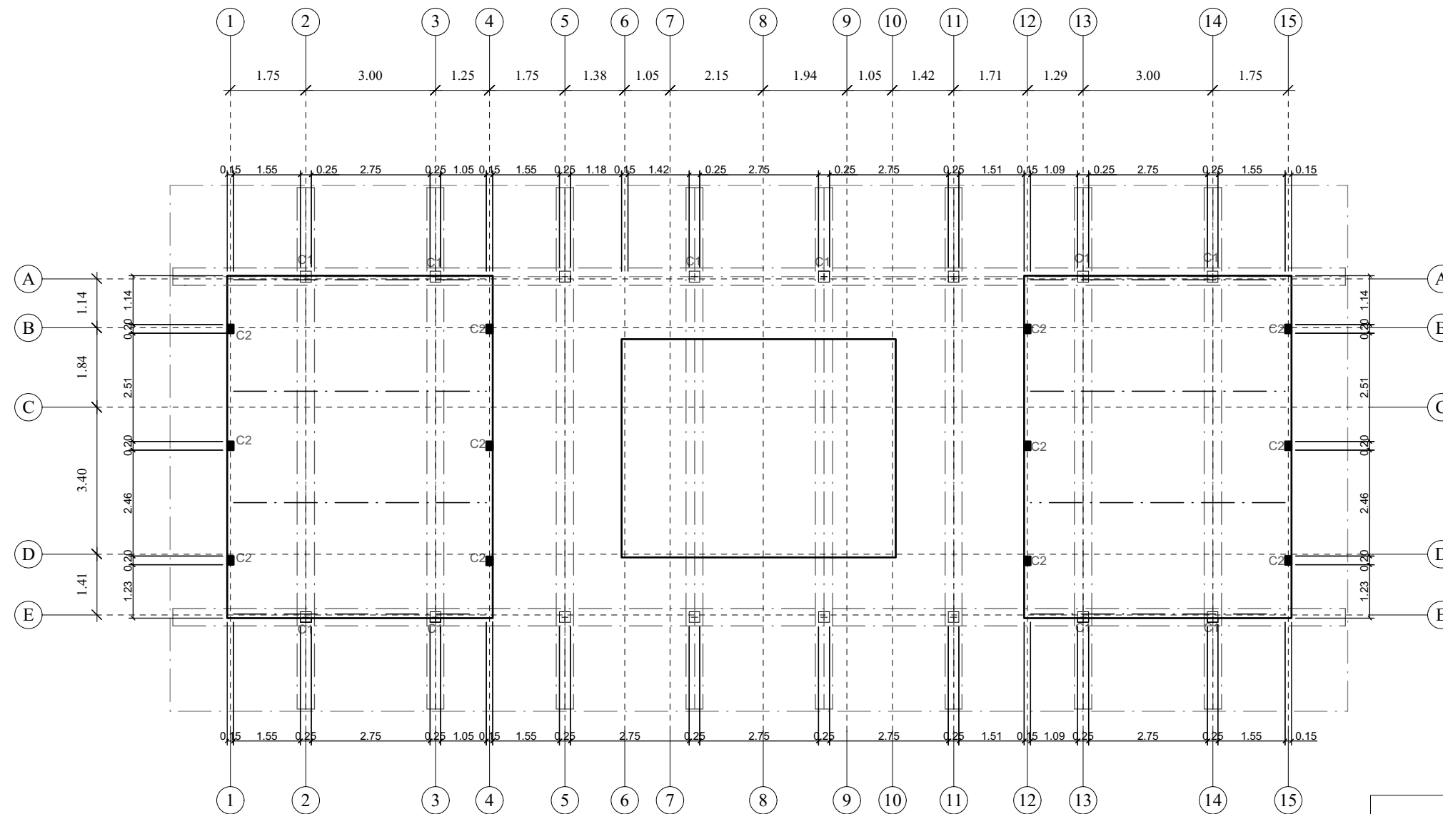
1 PLANTA ESTRUCTURAL DE TECHO Scale: 1:125
