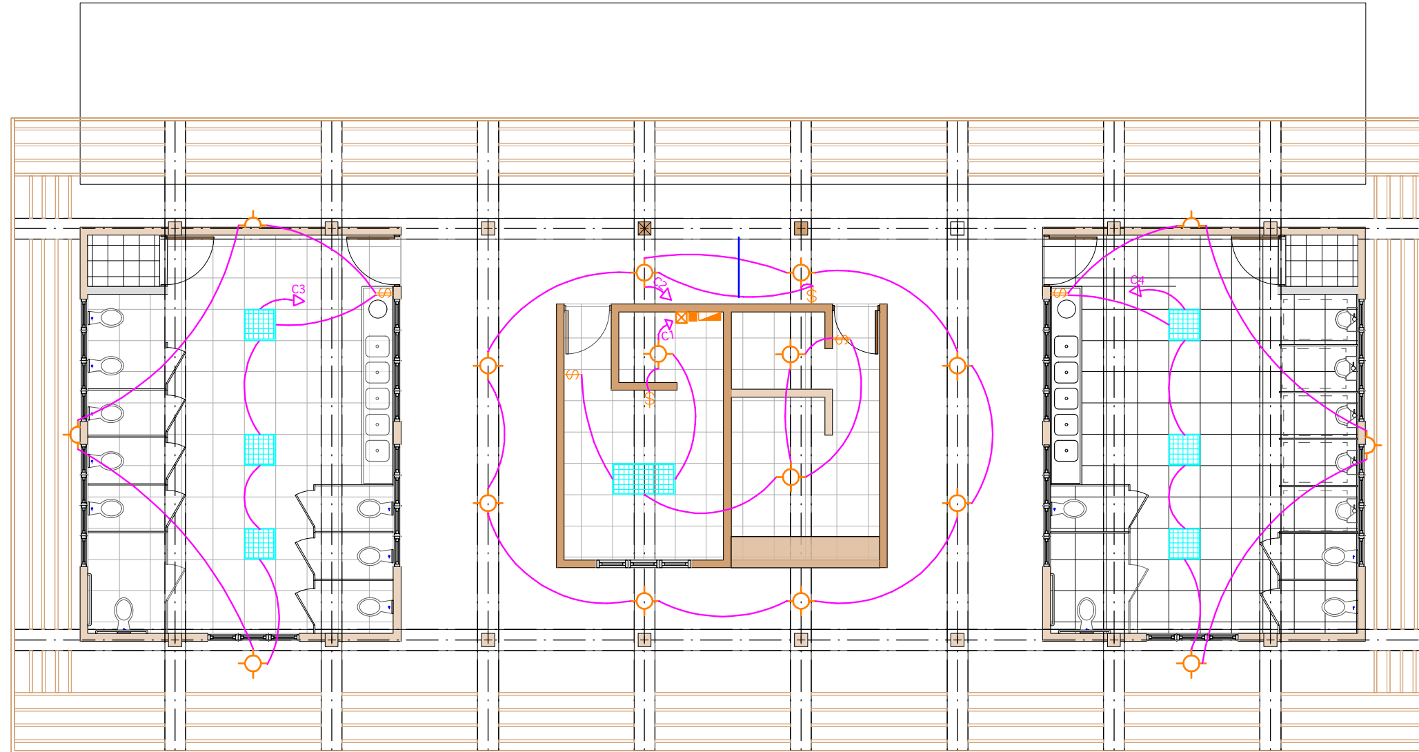
1 PLANTA DE LUMINARIA Scale: 1:100
