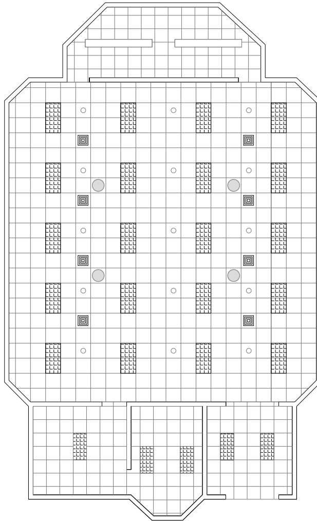
○ PLANTA DE PLAFOND ACTUAL No escala
