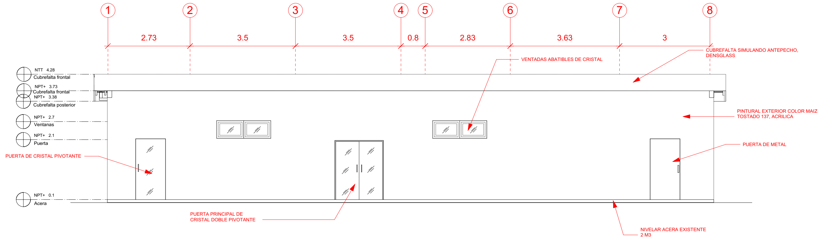
1 ELEVACION FRONTAL Scale: 1:75
