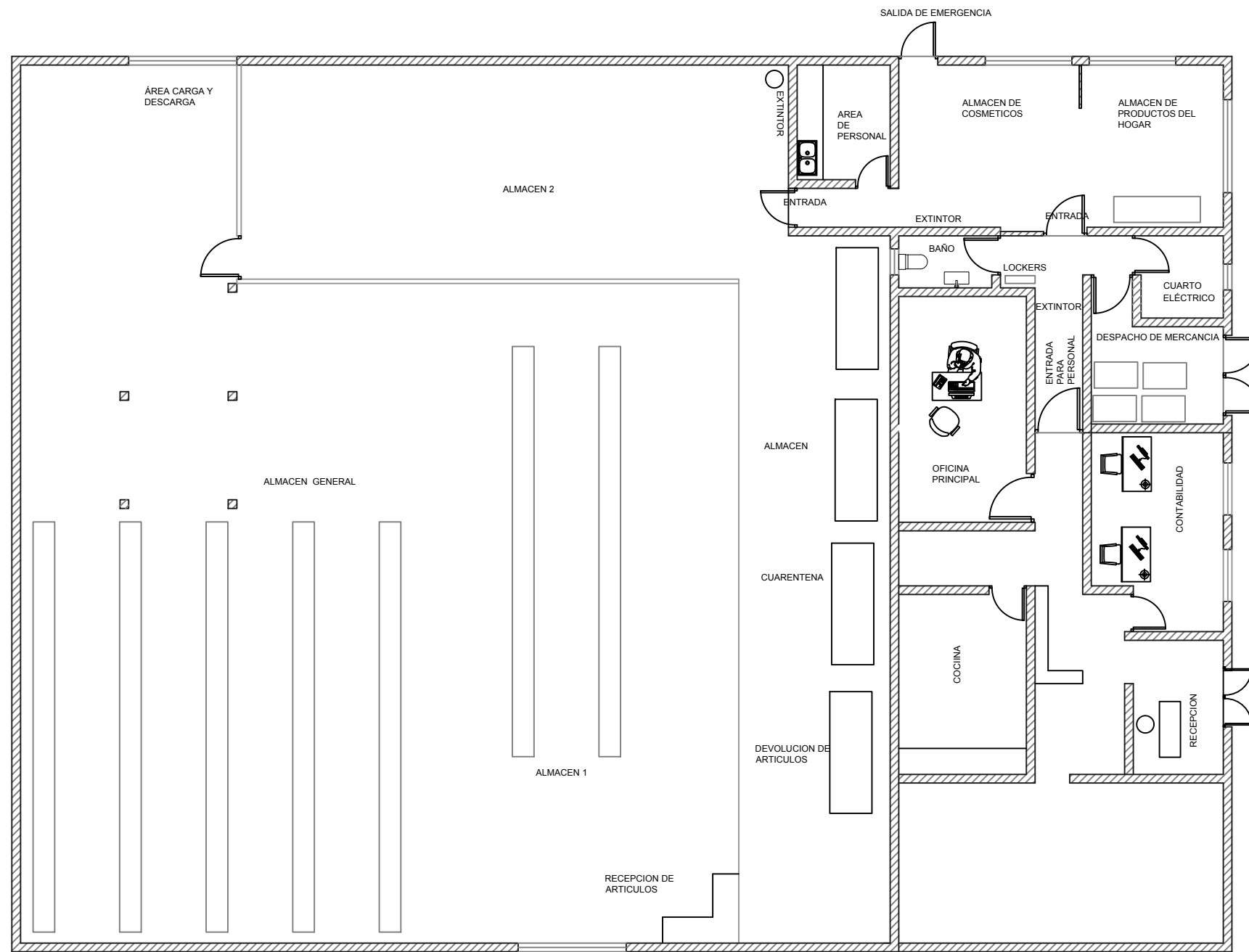
1.1 PLANTA ARQUITECTÓNICA AMUEBLADA UPSY MULTIMARCAS S.R.L. ESC:1:150
