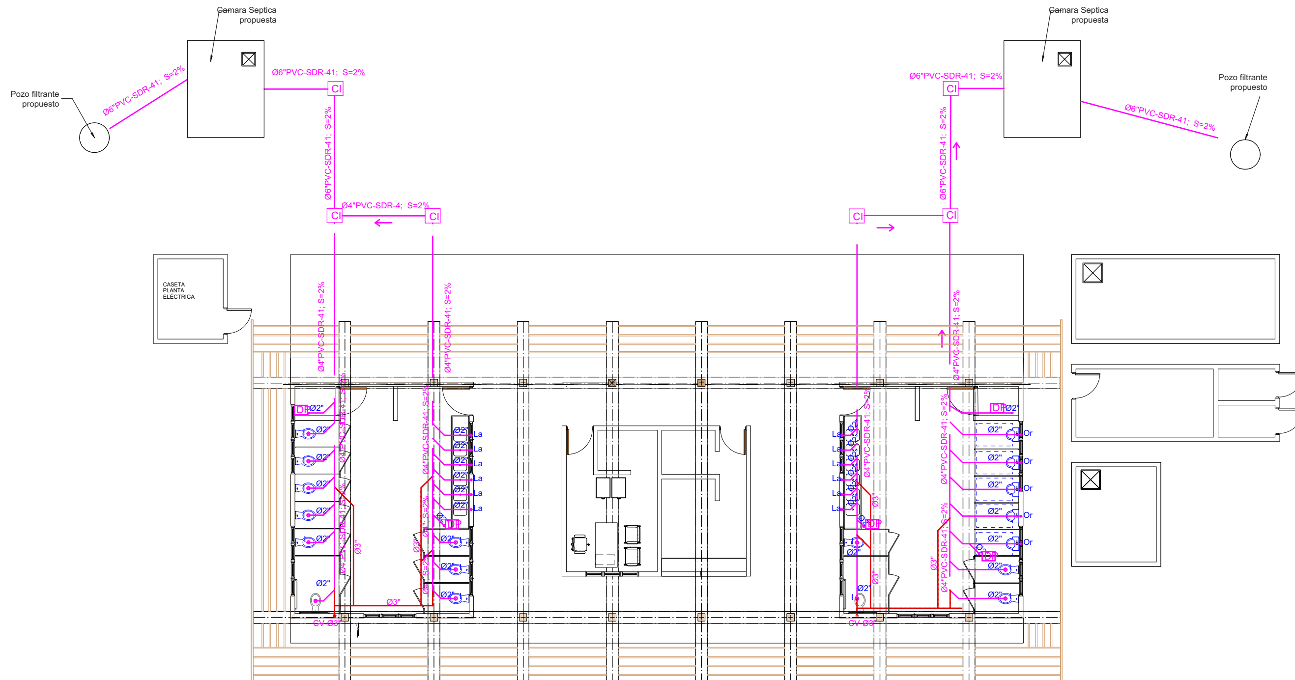
1 PLANTA SANITARIA - AGUAS NEGRAS Scale: 1:125
