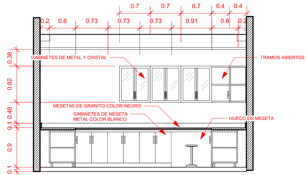
2 CORTE A-2 Scale: 1:50
