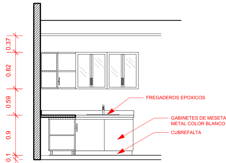
3 CORTE A-3 Scale: 1:50
