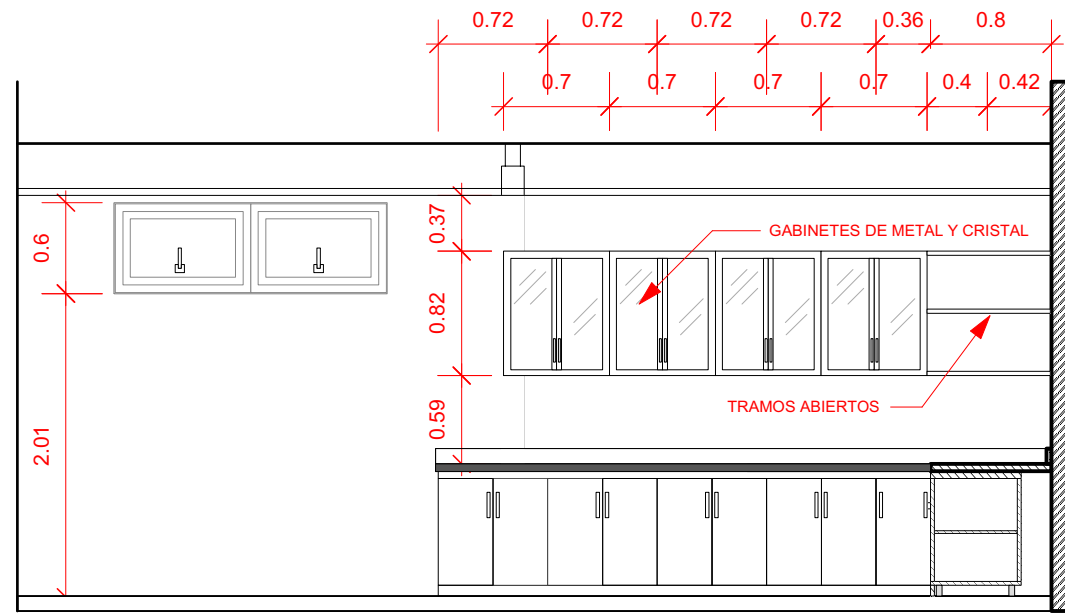
1 CORTE A-1 Scale: 1:50
